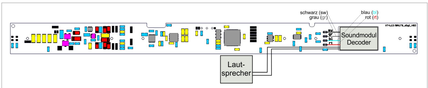
Abbildung 1: Montage SUSI-Soundmodul
