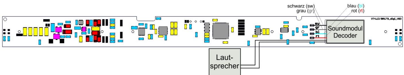
Abbildung 1: Montage SUSI-Soundmodul
